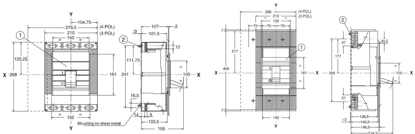
M3-630/AM3-800
