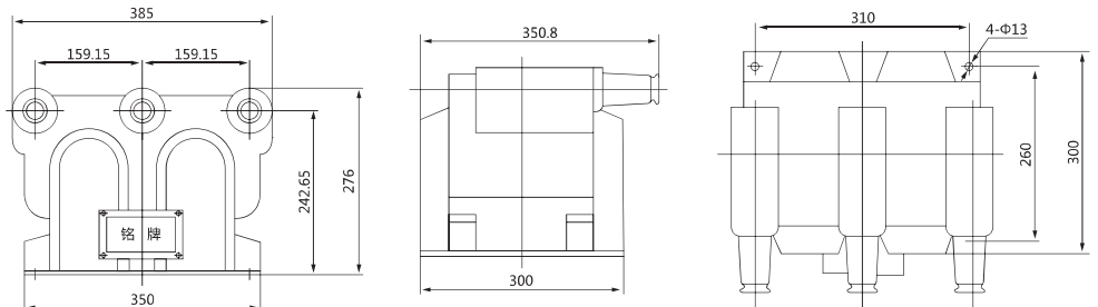
JSZV12-10R
