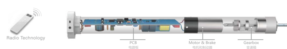
Inner Structure Picture 内部结构图
