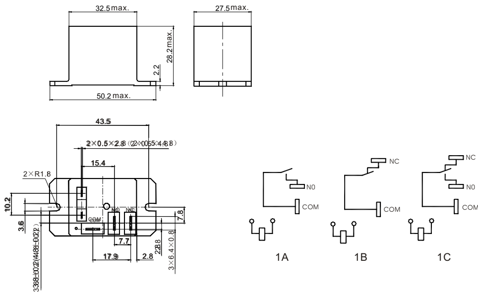
外形尺寸图
