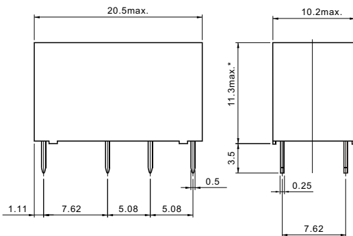
Dimensions
