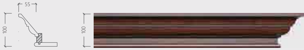
顶线：SD-1403 注：①此款顶线可调整高度，可做圆弧；②适用于橱柜、酒柜、书柜、衣柜、装饰柜、衣帽间；③H:100-150mm；④顶线外飘55mm。
