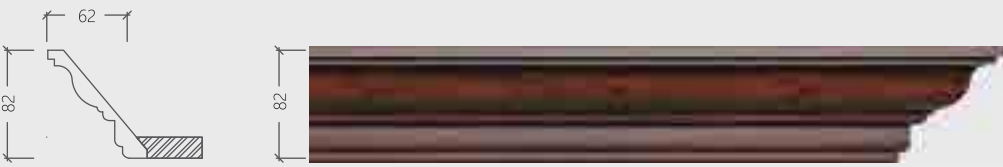
顶线：SD-0601 注：①此款顶线不可调整高度，不可做圆弧；②适用于橱柜、酒柜、书柜、衣柜、装饰柜、衣帽间。③顶线外飘62mm。
