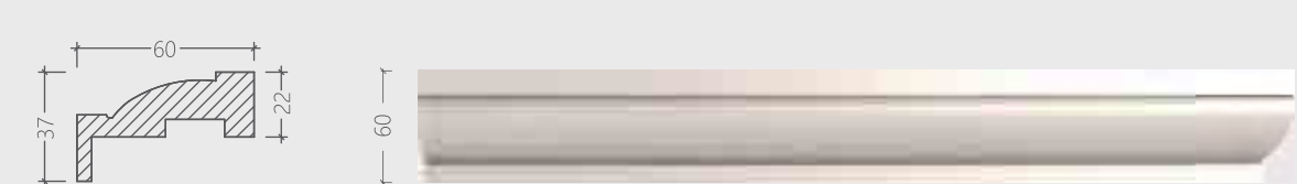
腰线：8#-S(T7#套线) 注：适用于门、窗、垭口、套线，护墙、背景墙压线
