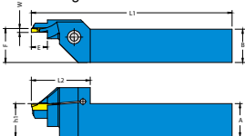
外徑端面刀架 External Grooving
