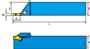
外徑切斷刀架 External Grooving
