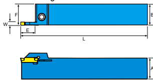
外徑切斷刀架 External Grooving
