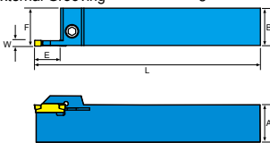
本圖所示為右手刀 (R) Right-Hand Show
