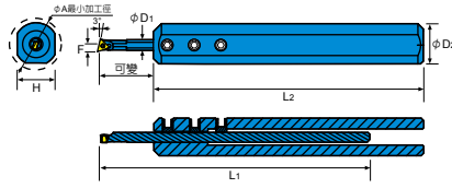
小徑內徑車刀架 Boring Bar
