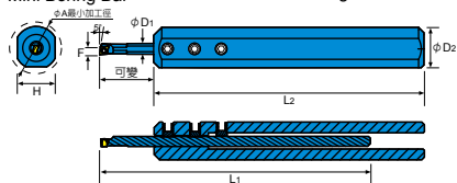
本圖所示為右手刀 (R) Right-Hand Show
