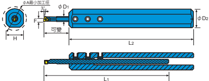
小徑內孔車刀架 Mini Boring Bar
