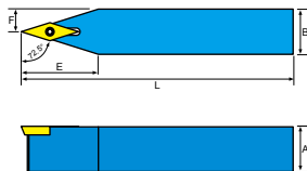
外徑車刀架
