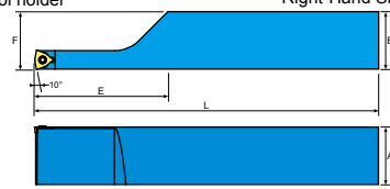
本圖所示為右手刀 (R) Right-Hand Show
