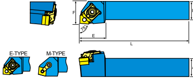
外徑車刀架 Tool holder
