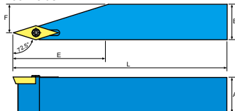
外徑車刀架
