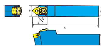
外徑車刀架 Tool holder
