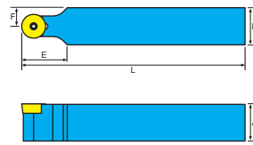
外徑車刀架 Tool holder
