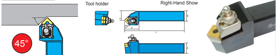
本圖所示為右手刀(R) Right-Hand Show
