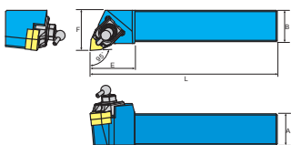
外徑車刀架 Tool holder
