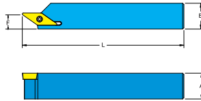
外徑車刀架 Tool holder
