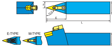
外徑車刀架 Tool holder
