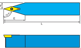
外徑車刀架 Tool holder
