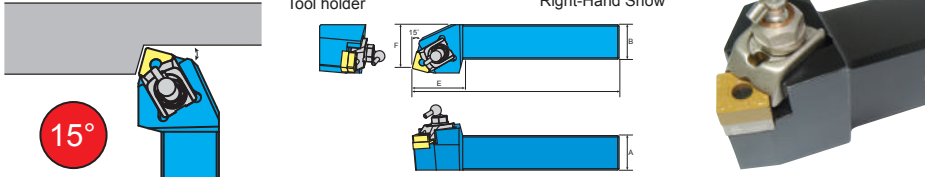
本圖所示為右手刀(R) Right-Hand Show
