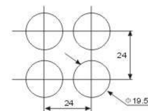
YHJ25安装尺寸 Install size
