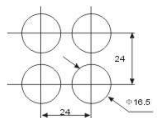
YHJ22安装尺寸 Install size
