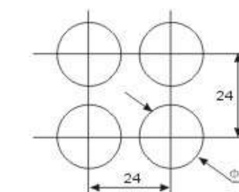
YHJ19安装尺寸 Install size
