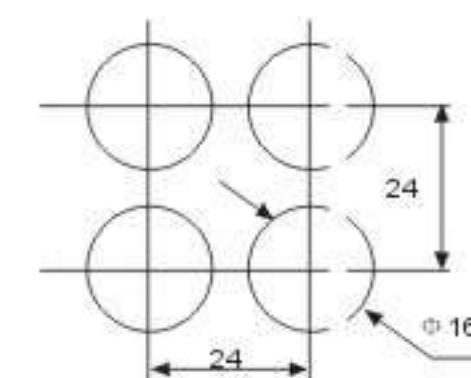
YHJ16安装尺寸 Install size
