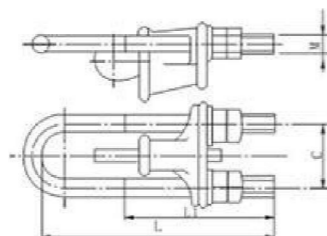
NUT线夹
