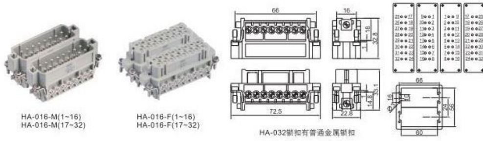
HA-032锁扣有普通金属锁扣
