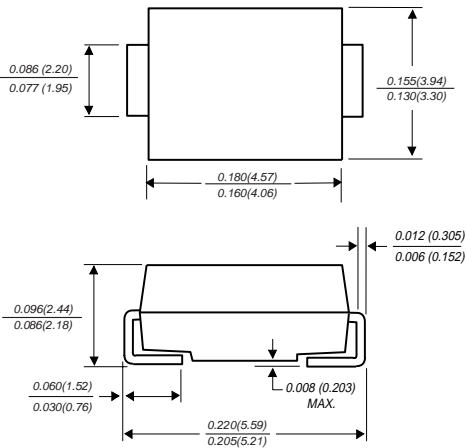
DO-214AA
